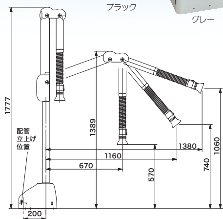
【寸法図】
